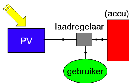
autonoom systeem
